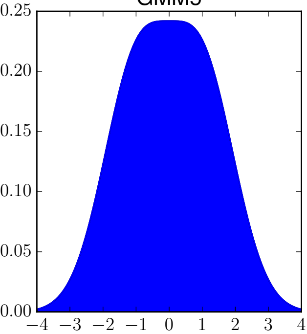
GMM5
