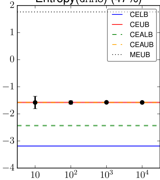
Entropy(GMM3) (47%)
