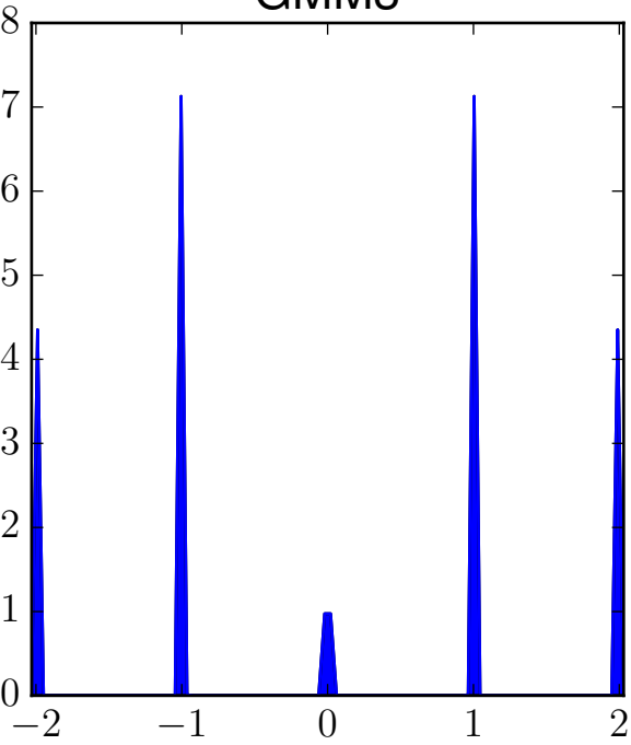
GMM3
