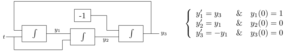
FIG. 3.2 – Génération de \cos et \sin par un GPAC : la version circuit est à gauche, et la version équation différentielle à droite. On a y_1 = \cos , y_2 = \sin , y_3 = -\sin .
