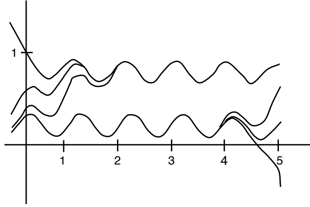
FIG. 2.4 – Quelques solutions de x' = 5x(1-x) - 0.8(1 + \sin(2\pi t)) .
